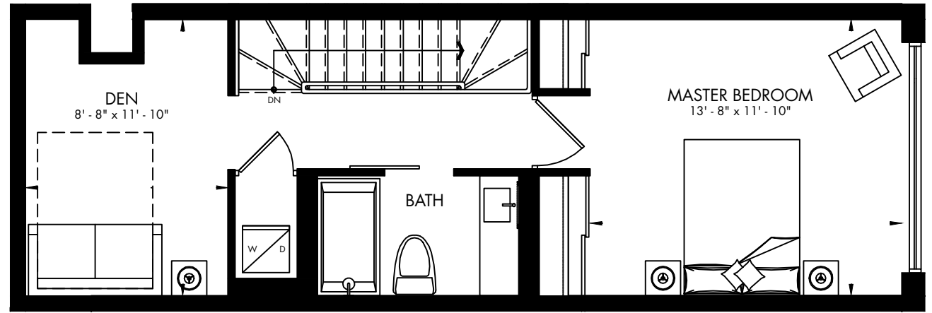
UPPER: INTERIOR 479 SQ.FT.
